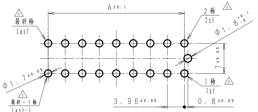
推奨基板レイアウト P.C.B Layout
