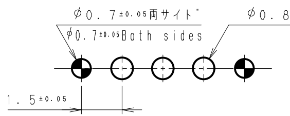
推奨基板レイアウト P.C.B. Layout
